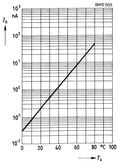
Dunkelstrom I_R = f(T_A) V_R = 5 \text{ V} , E = 0
