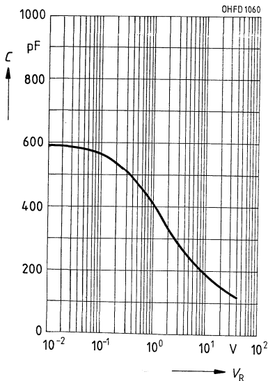
Kapazität C = f(V_R) f = 1 MHz, E = 0
