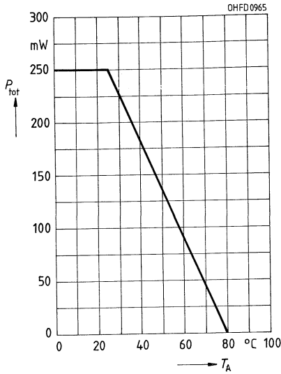
Verlustleistung P_{\text{tot}} = f(T_A)
