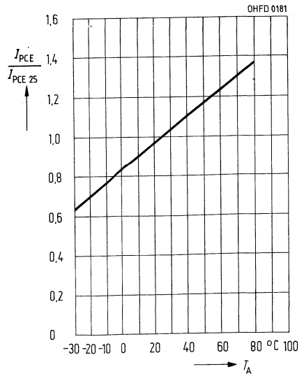
Fotostrom I_{PCE}/I_{PCE 25} = f(T_A) , V_{CE} = 5 V
