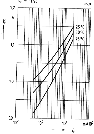
Vorwärtsspannung (typisch) der Diode V_F = f(I_F)
