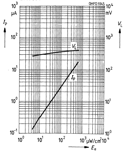
Fotostrom I_P = f(E_v) , V_R = 5\text{ V} Leerlaufspannung V_L = f(E_v) BPX 90 F
