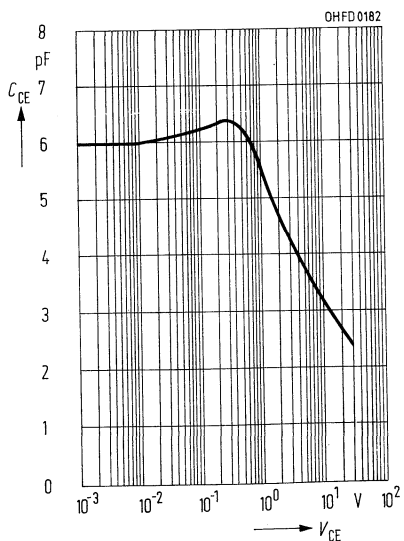
Kollektor-Emitter-Kapazität C_{\text{CE}} = f(V_{\text{CE}}) , f = 1 \text{ MHz} , E = 0
