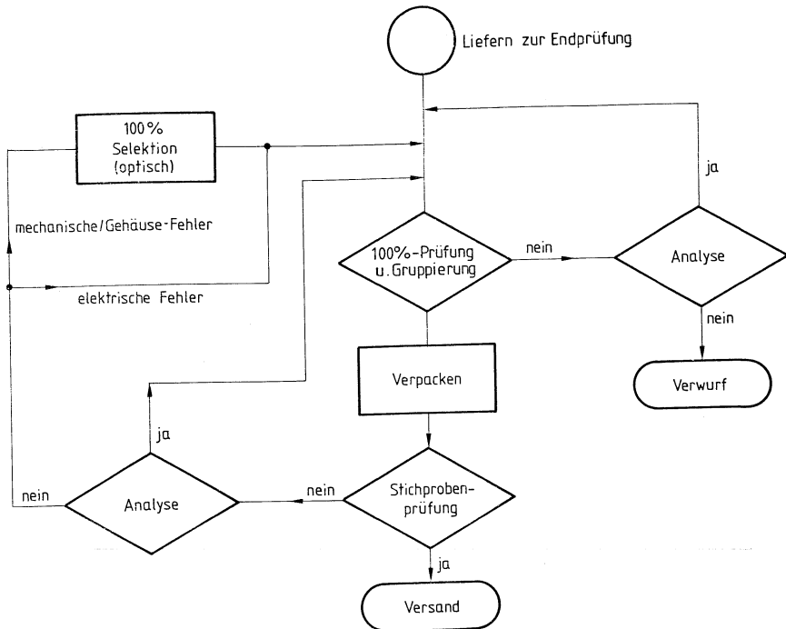
Bild 42 Ablaufdiagramm 100%-Endprüfung und Stichprobenprüfung
