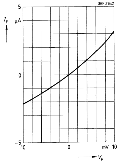
Nullpunktsteilheit I_F = f(V_F) E = 0
