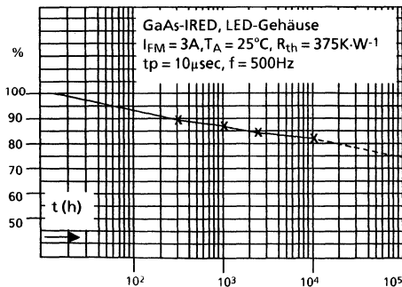
Bild 53 I_e = f(t)
