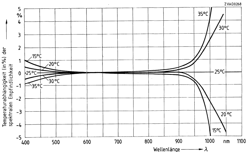
Bild 26 Temperaturabhängigkeit (in %) der spektralen Empfindlichkeit als Funktion der Wellenlänge bei PN-Fotodioden
