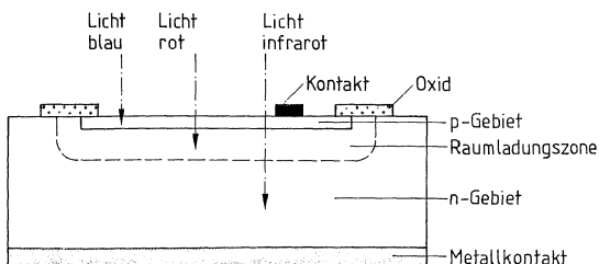
Bild 31 Fotodiode in Planartechnik
