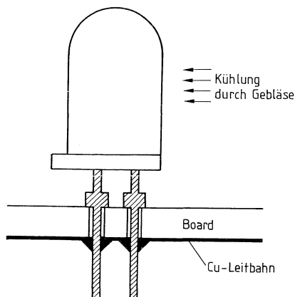
Bild 57 Günstigste Wärmeableitung durch – Abstand Chip – Lötstelle möglichst klein – Leitbahnen möglichst groß – zusätzliche Luftkühlung
