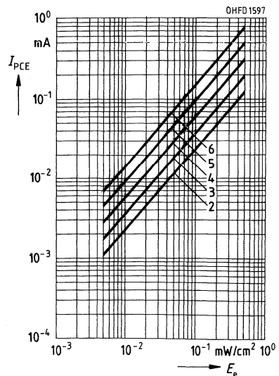
Fotostrom I_{PCE} = f(E_e) V_{CE} = 5 \text{ V}
