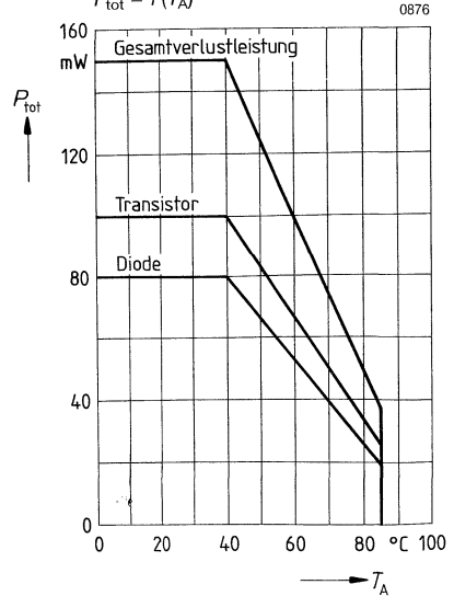
Zulässige Verlustleistung für Diode und Transistor P_{tot} = f(T_A)
