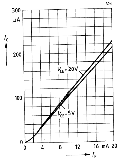
Kollektorstrom, I_C = f(I_F) Abstand d zum Reflektor = 1 mm, 90% Reflexion
