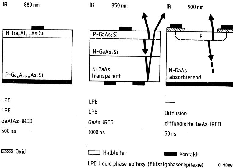
Bild 7 Aufbau der Diodenkörper für IRED
