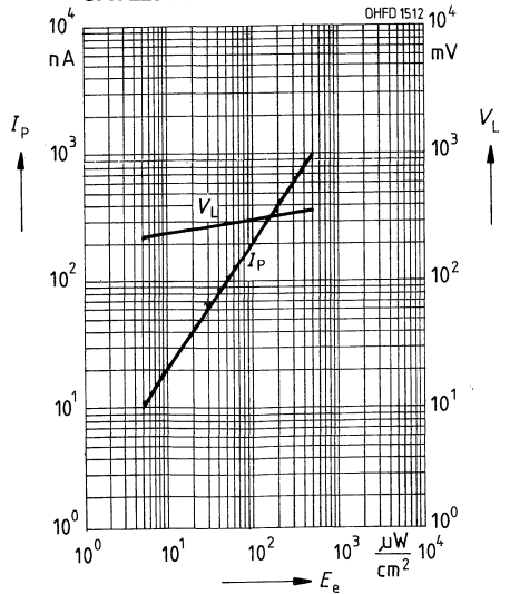
Fotostrom I_P = f(E_e) , V_R = 5\text{ V} Leerlaufspannung V_L = f(E_e) SFH 229 PF
