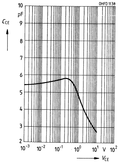
Kollektor-Emitter-Kapazität
