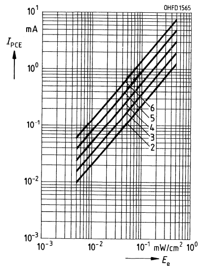
Fotostrom I_{PCE} = f(E_e)
