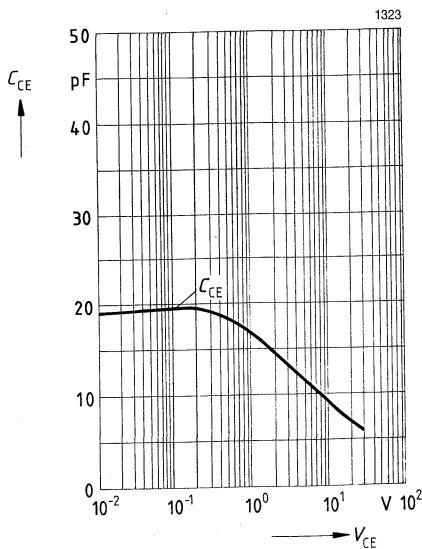
Transistor-Kapazität (typisch), C_{CE} = f(V_{CE}) T_A = 25 \text{ }^\circ\text{C} , f = 1 \text{ MHz}
