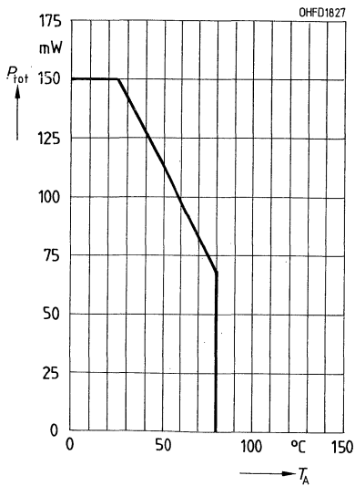
Verlustleistung P_{tot} = f(T_A) KOM 2033 B, KOM 2100 B
