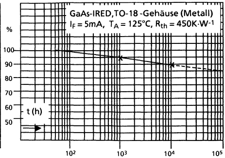
Bild 56 I_e = f(t)
