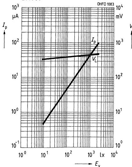
Fotostrom I_P = f(E_v) , V_R = 5\text{ V} Leerlaufspannung V_L = f(E_v) BPX 90
