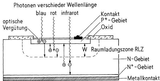
Bild 1 Planare Si-Fotodiode (Schema)
