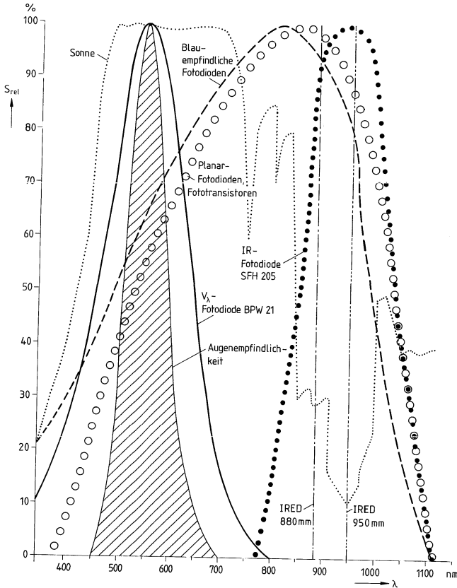
Bild 30 Wellenlängendiagramm
