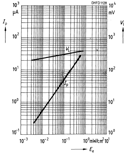
Fotostrom I_p = f(E_e) , V_R = 5\text{ V} Leerlaufspannung V_L = f(E_e) SFH 2030 F
