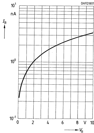
Dunkelstrom I_R = f(V_R)
