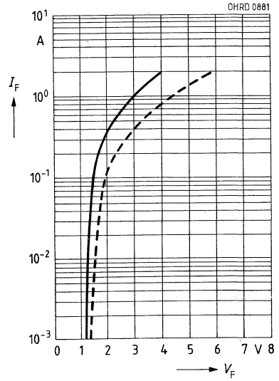
Durchlaßstrom I_F = f(V_F) Einzelpuls, \tau = 20 \mu\text{s}
