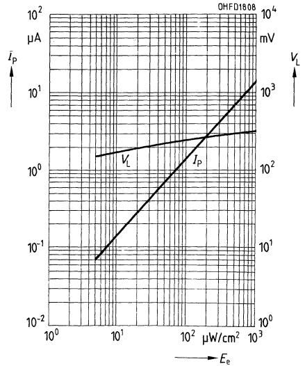
Fotostrom I_P = f(E_e) , V_R = 5 V Leerlaufspannung V_L = f(E_e) BPX 48 F
