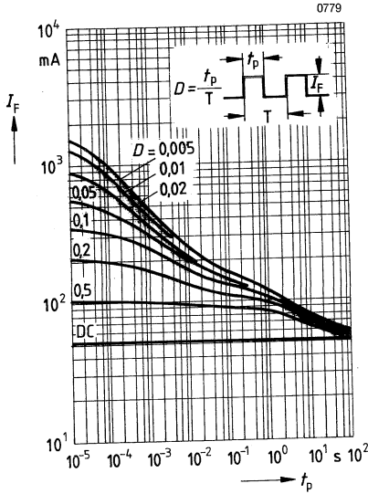
Zulässige Impulsbelastbarkeit, I_F = f(t_p) D = \text{Parameter, } T_A = 25^\circ\text{C}
