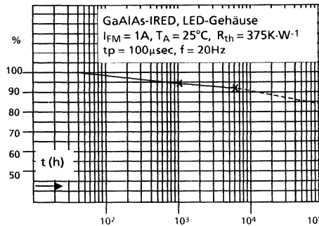
Bild 45 I_e = f(t)
