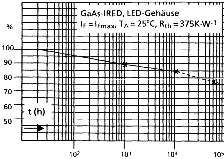
Bild 49 I_e = f(t)
