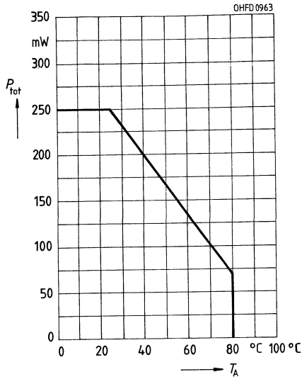
Verlustleistung P_{\text{tot}} = f(T_A)
