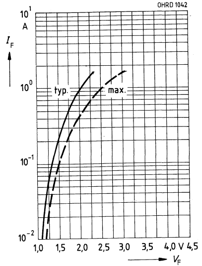
Durchlaßstrom I_F = f(V_F) Einzelpuls, \tau = 20 \mu s
