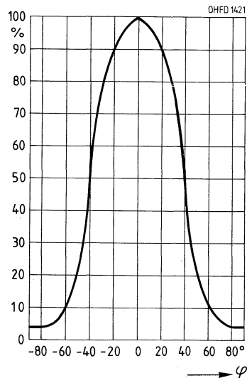
Richtcharakteristik
