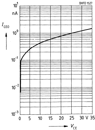
Dunkelstrom I_{\text{CEO}} = f(V_{\text{CE}}) E = 0
