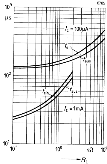
Schaltzeiten t = f(R_L) T_A = 25^\circ\text{C}, I_F = 10\text{ mA}
