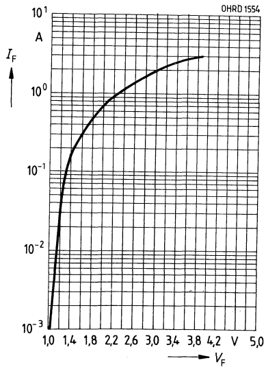
Durchlaßstrom I_F = f(V_F) Einzelpuls, \tau = 20 \mu s
