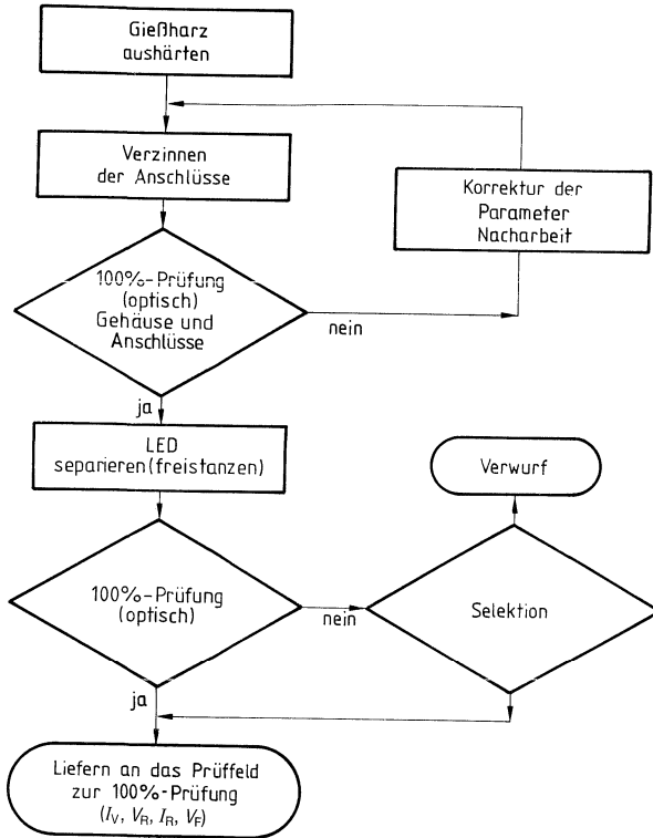
Bild 41 Ablaufdiagramm IRED-Produktion in LED-Bauform
