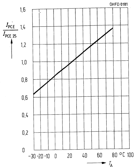
Fotostrom I_{\text{PCE}}/I_{\text{PCE}25} = f(T_A) , V_{\text{CE}} = 5 \text{ V}
