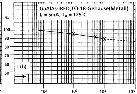
Bild 48 I_e = f(t)
