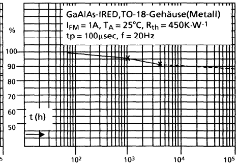
Bild 46 I_e = f(t)
