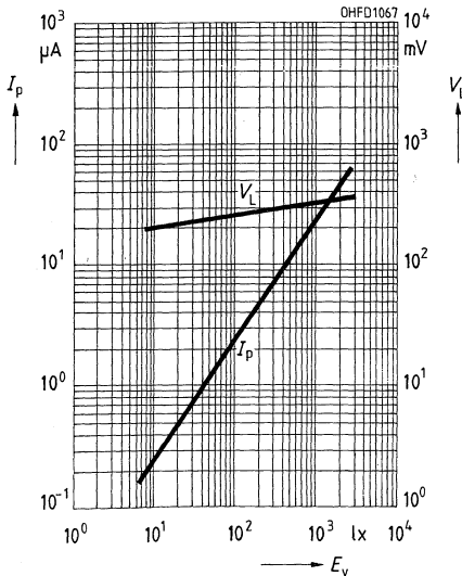
Fotostrom I_P = f(E_v) , V_R = 5 V Leerlaufspannung V_L = f(E_v) BPX 48
