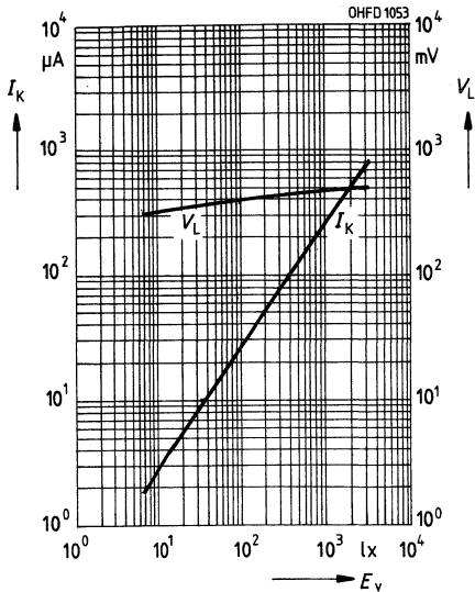
Leerlaufspannung V_L = f(E_v) Kurzschlussstrom I_K = f(E_v)
