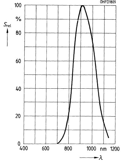
Relative spektrale Empfindlichkeit BPX 48 F
