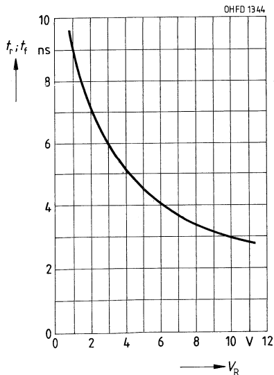
Schaltzeiten t_r/t_f = f(V_R) R_L = 50 \Omega
