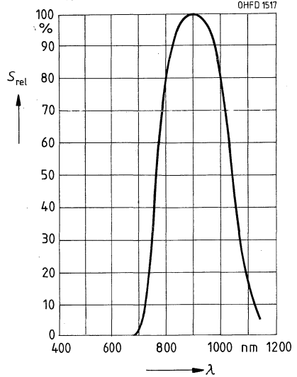
Relative spektrale Empfindlichkeit SFH 229 PF
