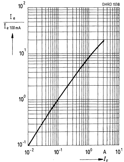
Rel. Strahlstärke \frac{I_e}{I_{e 100 \text{ mA}}} = f(I_F)
