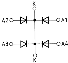
Schaltbild
