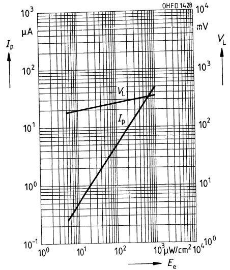
Fotostrom I_p = f(E_e) , V_R = 5\text{ V} Leerlaufspannung V_L = f(E_e)
