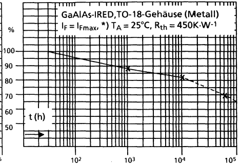
Bild 44 I_e = f(t)
