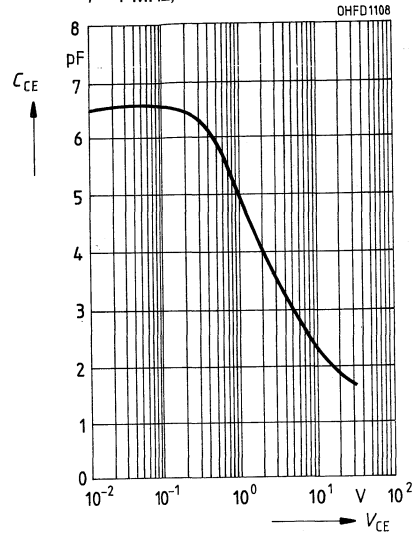
Kollektor-Emitter-Kapazität C_{CE} = f(V_{CE}) , f = 1\text{ MHz}, E = 0
