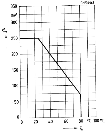
Verlustleistung P_{\text{tot}} = f(T_A)
