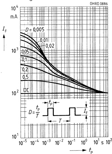
Zulässige Impulsbelastbarkeit I_F = f(t, T_A = 25^\circ\text{C}) , Tastgrad D = \text{Parameter}
