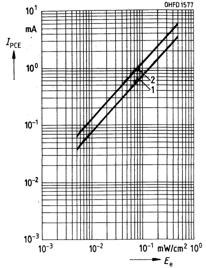
Fotostrom I_{PCE} = f(E_e) V_{CE} = 5 V
