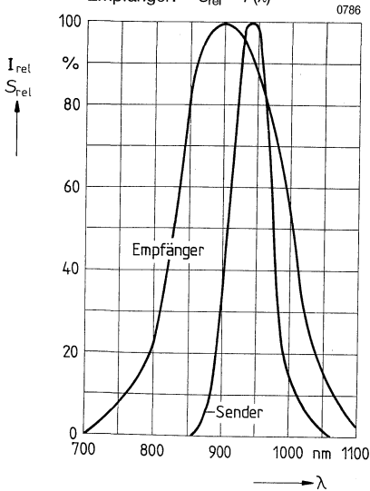
Relative spektrale Verteilung vom Sender (GaAs) und Empfänger (Si)
