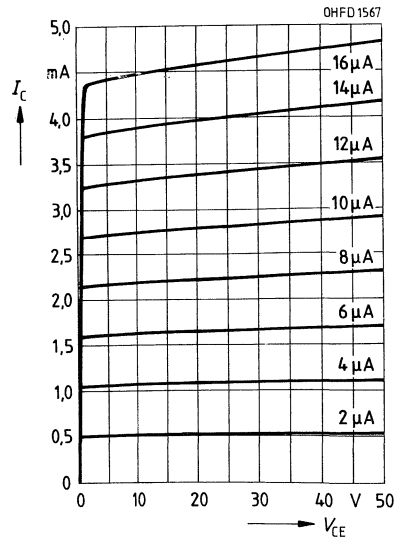
Ausgangskennlinien I_C = f(V_{CE}) I_B = \text{Parameter}
