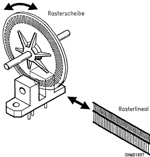
Bild 2 Gabellichtschranke
