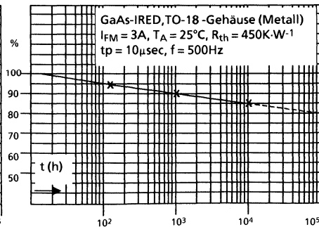
Bild 54 I_e = f(t)
