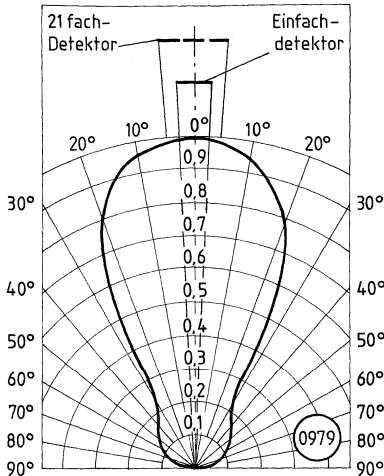
Bild 20 Idealisierte Anstrahlcharakteristik der LD 271
