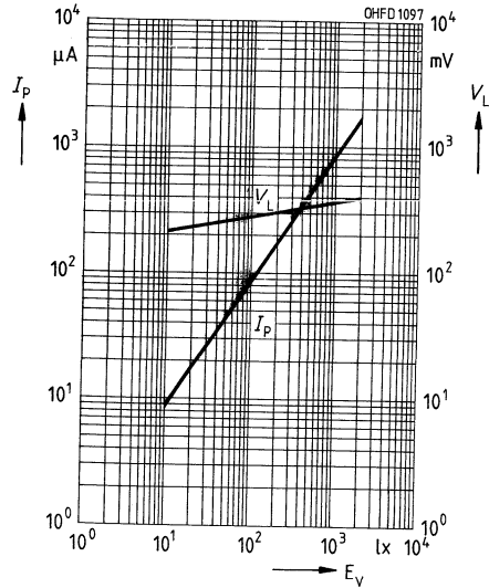
Fotostrom I_P = f(E_V) , V_{R1} = 5\text{ V} Leerlaufspannung V_L = f(E_V)
