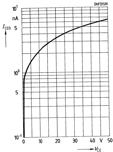
Dunkelstrom I_{CEO} = f(V_{CE}) E = 0
