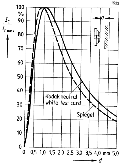
Kollektorstrom \frac{I_C}{I_{C \max}} = f(d)
