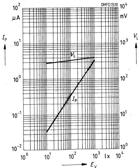
Fotostrom I_P = f(E_V) , V_R = 5\text{ V} Leerlaufspannung V_L = f(E_V) SFH 229 P
