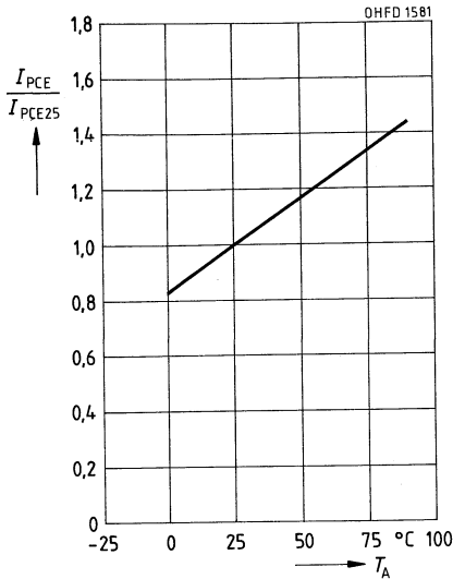
Fotostrom I_{PCE}/I_{PCE25} = f(T_A) V_{CE} = 5 \text{ V}
