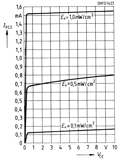
Fotostrom I_{PCE} = f(V_{CE}) Parameter E_e
