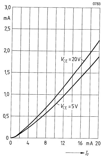
Kollektorstrom, I_C = f(I_F) Abstand d zum Reflektor = 1 mm, 90% Reflexion
