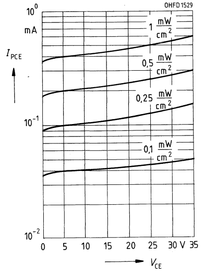
Fotostrom I_{\text{PCE}} = f(V_{\text{CE}}) E_c = \text{Parameter}
