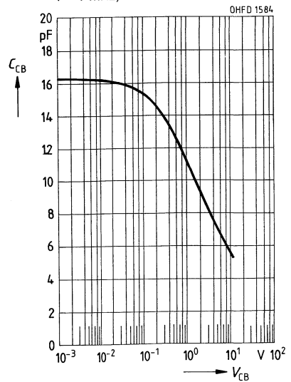
Kollektor-Basis-Kapazität C_{CB} = f(V_{CB}) f = 1 \text{ MHz}, E = 0
