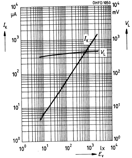
Leerlaufspannung V_L = f(E_v) Kurzschlußstrom I_K = f(E_v)
