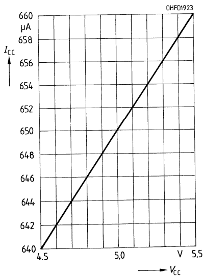
Stromaufnahme I_{CC} = f(V_{CC})
