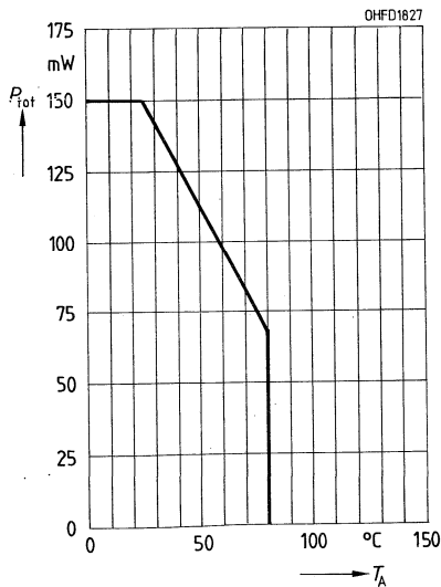
Verlustleistung P_{tot} = f(T_A) KOM 2033 A, KOM 2100 A
