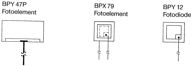
Bild 34 Beispiele für offene Bauform
