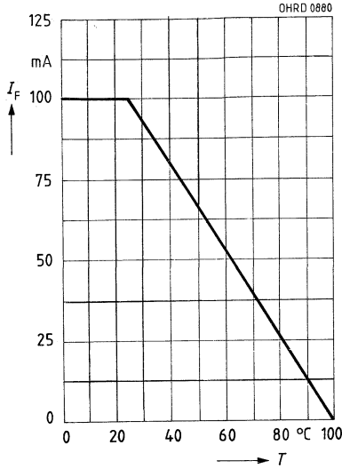
Maximal zulässiger Durchlaßstrom I_F = f(T_A)
