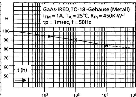
Bild 52 I_e = f(t)
