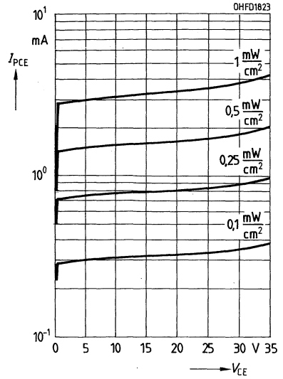
Fotostrom I_{\text{PCE}} = f(V_{\text{CE}}) E_0 = \text{Parameter}
