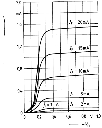
Ausgangskennlinien (typisch), I_C = f(V_{CE}) Abstand zum Reflektor: d = 1 \text{ mm} , 90% Reflexion, T_A = 25 \text{ }^\circ\text{C}
