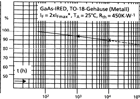
Bild 50 I_e = f(t)
