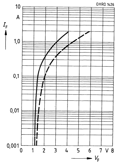
Durchlaßstrom I_F = f(V_F)
