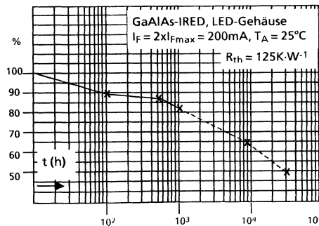
Bild 47 I_e = f(t)
