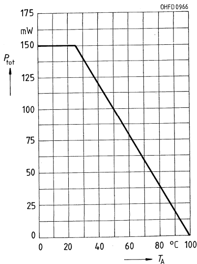
Verlustleistung P_{tot} = f(T_A)
