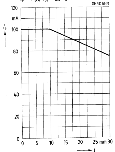
Max. Durchlaßstrom in Abhängigkeit von der freien Beinchenlänge I_F = f(l) , T_A = 25^\circ\text{C}
