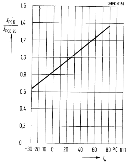
Fotostrom I_{PCE}/I_{PCE25} = f(T_A) , V_{CE} = 5\text{ V}
