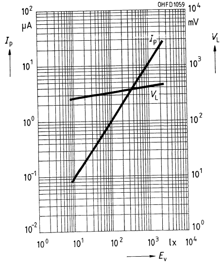
Fotostrom I_P = f(E_v) , V_R = 5 \text{ V} Leerlaufspannung V_L = f(E_v)
