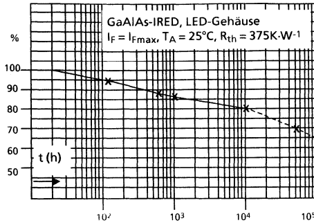
Bild 43 I_e = f(t)
