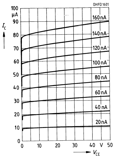
Ausgangskennlinien I_C = f(V_{CE}) I_B = Parameter
