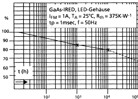
Bild 51 I_e = f(t)
