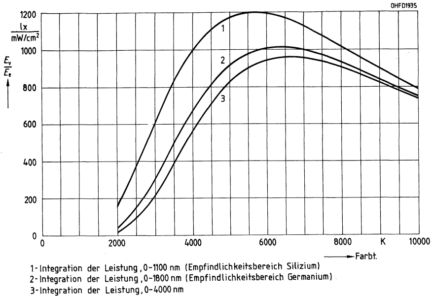
Bild 24 Umrechnung der Beleuchtungsstärke E_v in Bestrahlungsstärke E_e . Schwarzer Planckscher Strahler als Funktion der Farbtemperatur.
