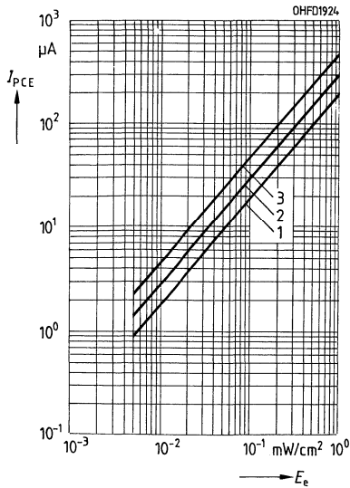
Fotostrom I_{PCE} = f(E_e) V_{CE} = 5 V
