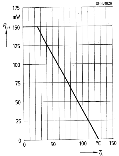
Verlustleistung P_{tot} = f(T_A) KOM 2033 AF, KOM 2100 AF
