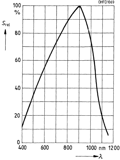
Relative spektrale Empfindlichkeit BPX 48
