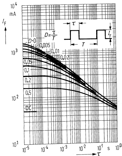
Zulässige Impulsbelastbarkeit I_F = f(\tau) , T_C = 25^\circ C , Tastgrad D = \text{Parameter}
