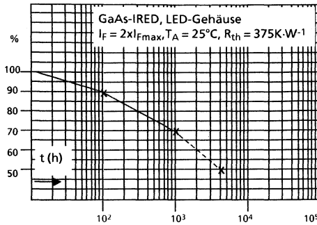
Bild 55 I_e = f(t)
