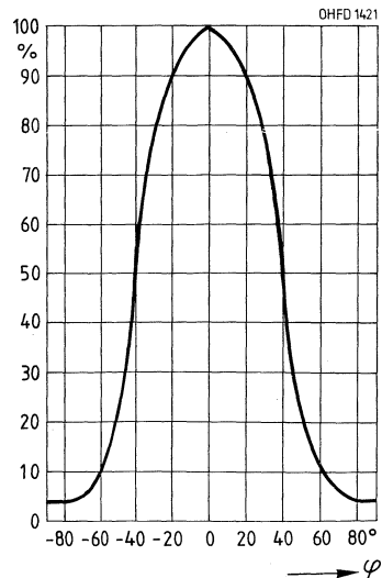
Richtcharakteristik
