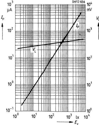
Fotostrom I_p = f(E_v) , V_R = 5\text{ V} Leerlaufspannung V_L = f(E_v) SFH 2030
