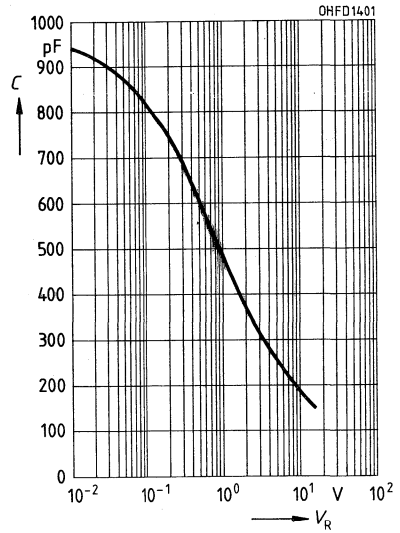
Kapazität C = f(V_R) f = 1 \text{ MHz}, E = 0
