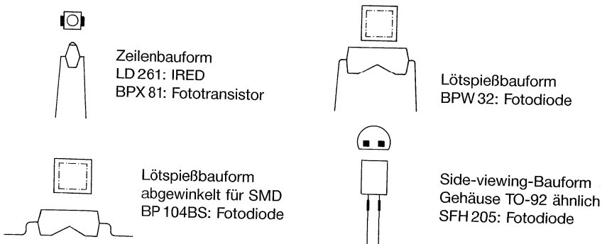
Bild 35 Beispiele für Lötspießbauformen und Side-viewing-Bauform
