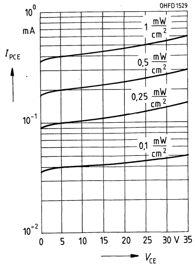
Fotostrom I_{PCE} = f(V_{CE}) E_0 = \text{Parameter}
