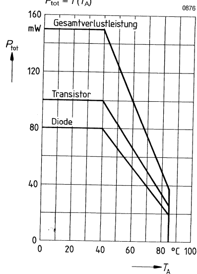
Zulässige Verlustleistung für Diode und Transistor P_{\text{tot}} = f(T_A)
